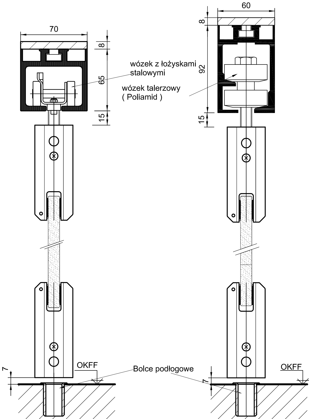
Szyna ALU Typ L
